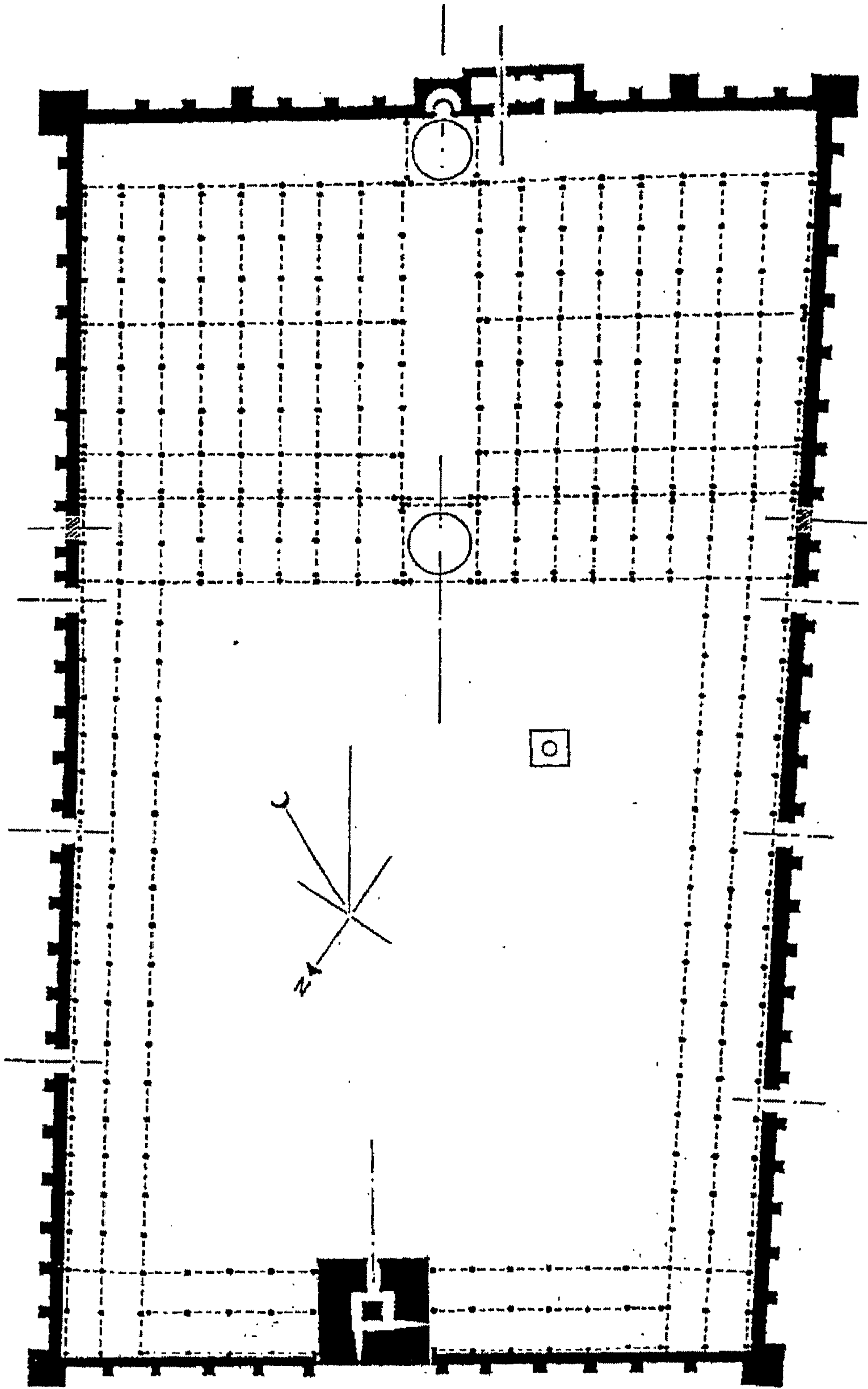
(شكل رقم ١٠) رسم تخطيطي لجامع القيروان في عهد ابراهيم بن احمد عن ليزين
